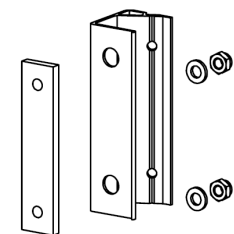
Väggfäste till gejder
